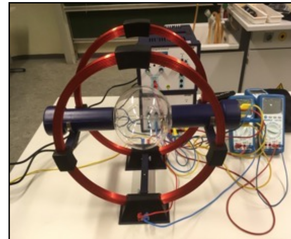
Versuchsaufbau Physik
